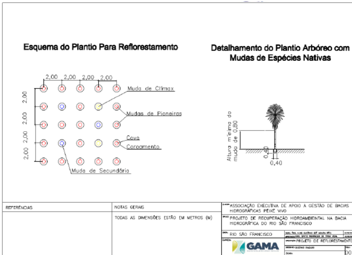
Figura 21: Especificações técnicas para execução do plantio das mudas nas áreas das subbacias da UTE Guaicuí
