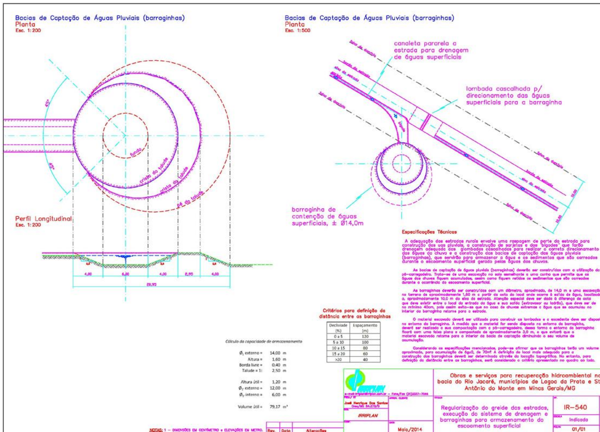
Figura 17: Layout com especificações técnicas para a construção de barraginhas para drenagem de estradas rurais
